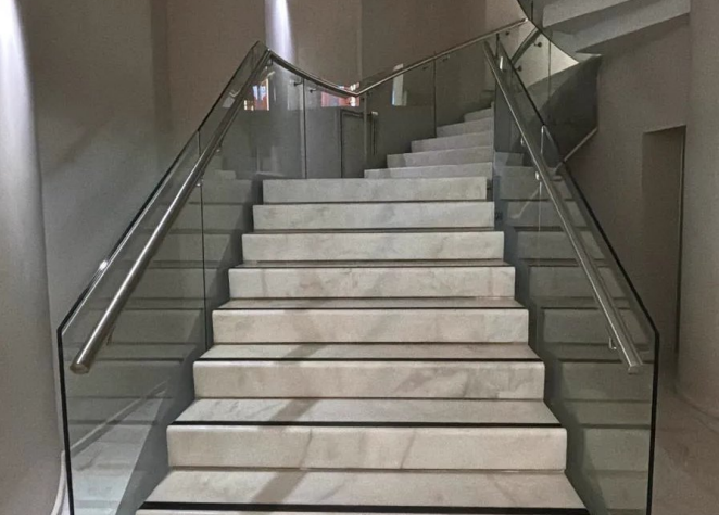
Paslanmaz Korkuluk Modeli 01 | FK-PK-01
